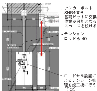
ホールダウン金物柱脚部
