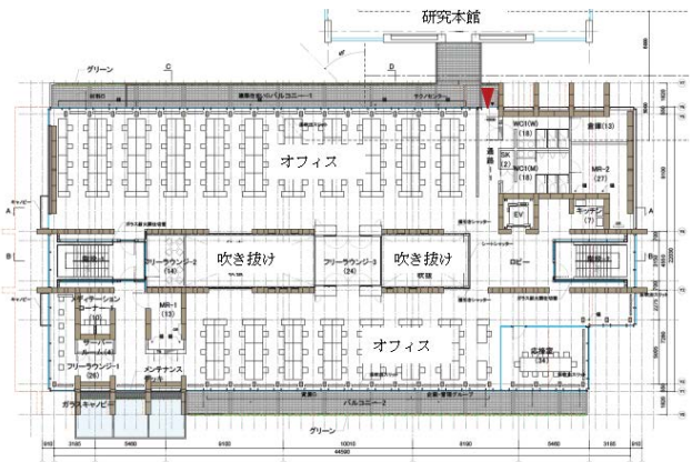
2階平面図
