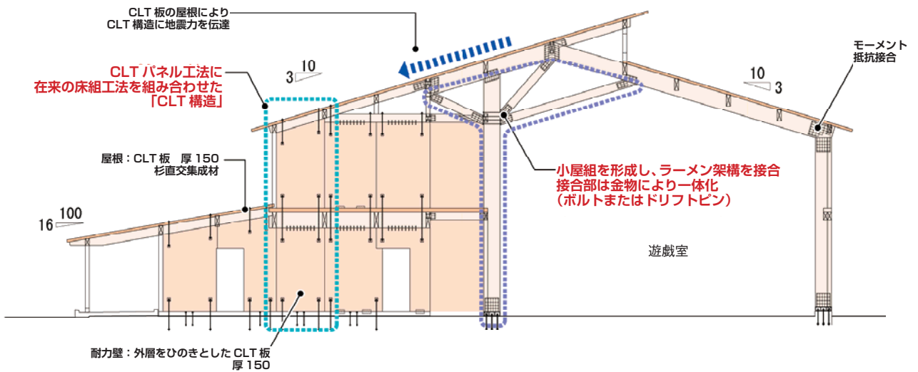
機能性と安全性を確保したハイブリッド架構形式
