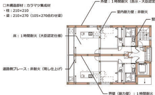
3, 4 階平面図
