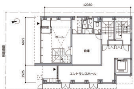
1 階平面図
