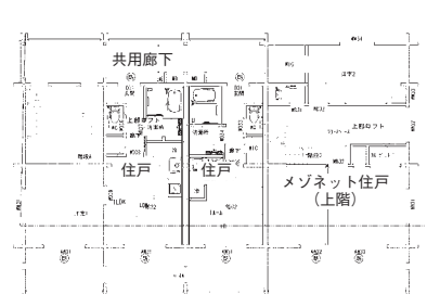
3階平面図
