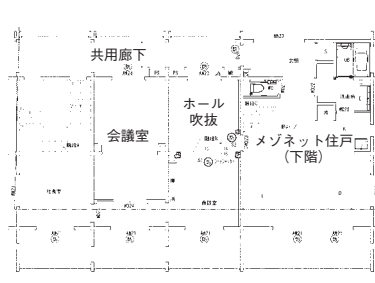
2階平面図
