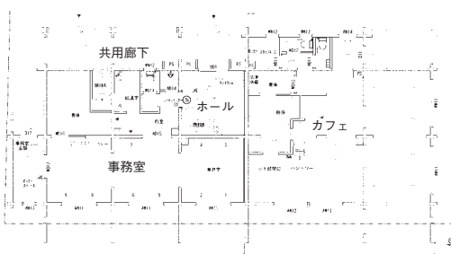
1階平面図
