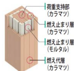
3層式の耐火集成材を採用
