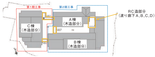
配置計画図
