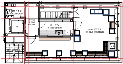
10階平面図
