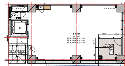
4~6階平面図
