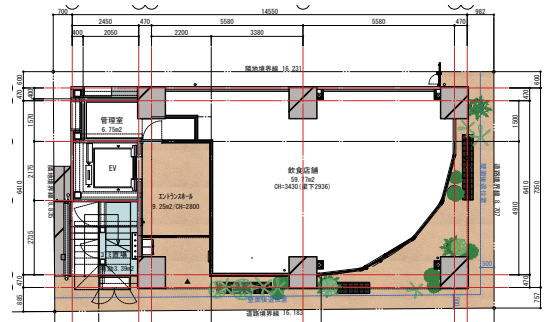
1階平面図
