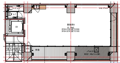
2~3階平面図
