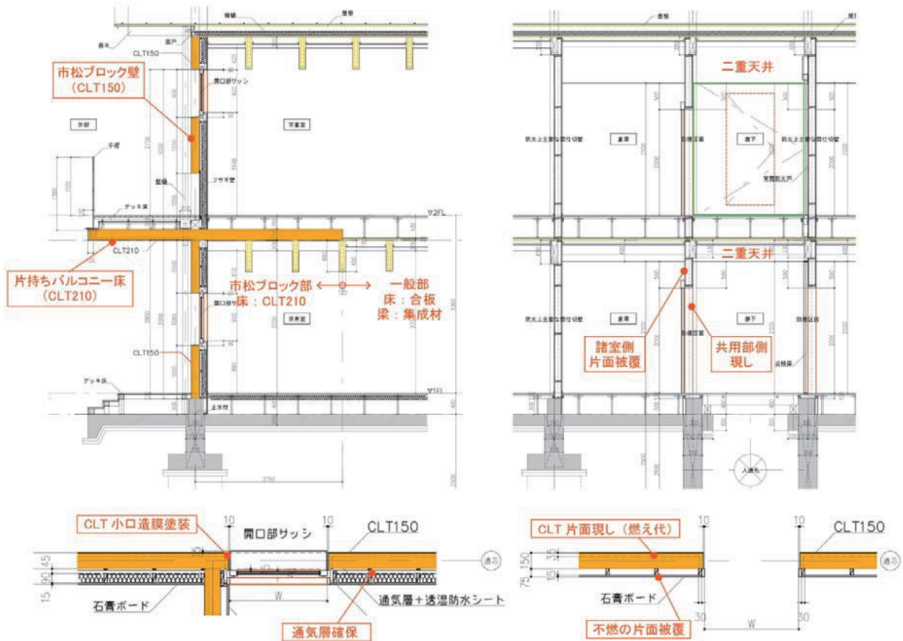
各部詳細図
