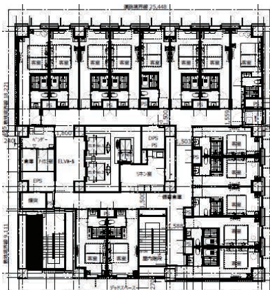
5~8階平面図
