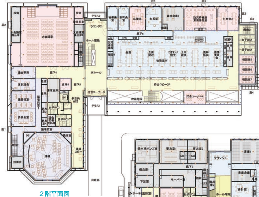
2階平面図
