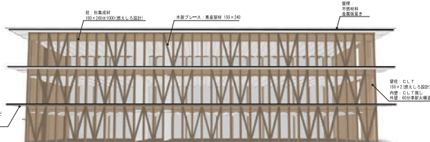
北面ファサード
