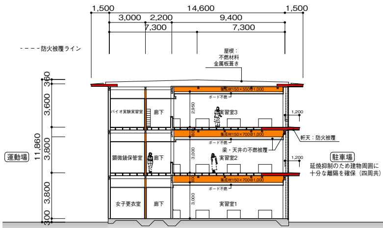
断面図
