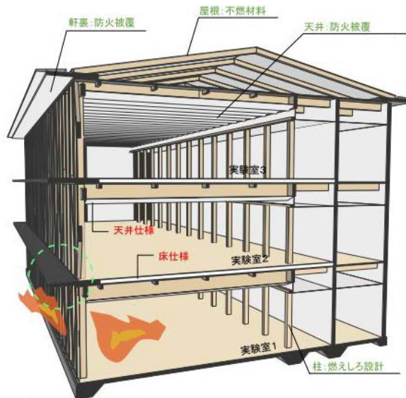
CLT底による上階への延焼抑制
