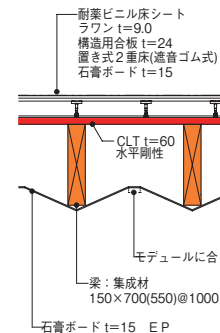
天井・床構造の仕様
