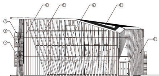
東側立面図
