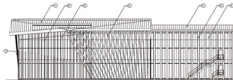
北側立面図
