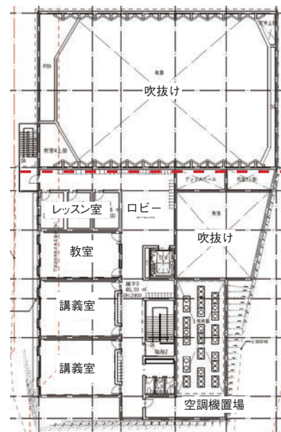
3階平面図
