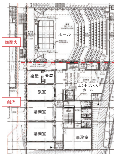
1階平面図
