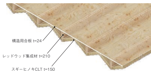
CLT 折版部のイメージ
