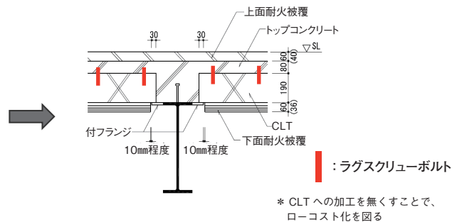
CLT と鉄骨梁の簡易な接合方法を開発
