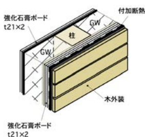
木造耐火構造壁
