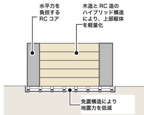
構造計画の考え方
