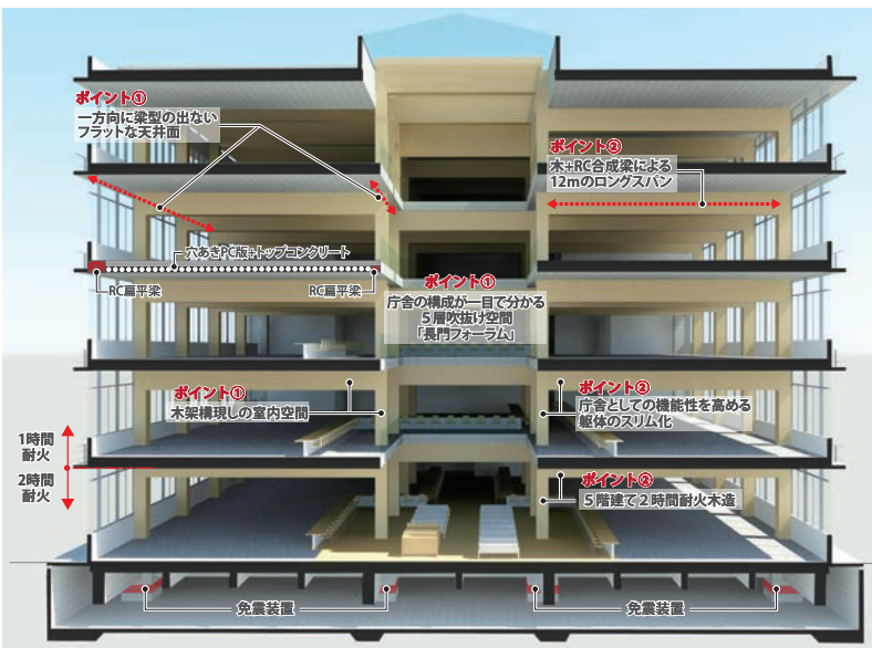
断面イメージ (A-A' 断面)
