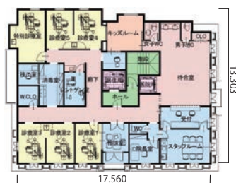
2階平面図
