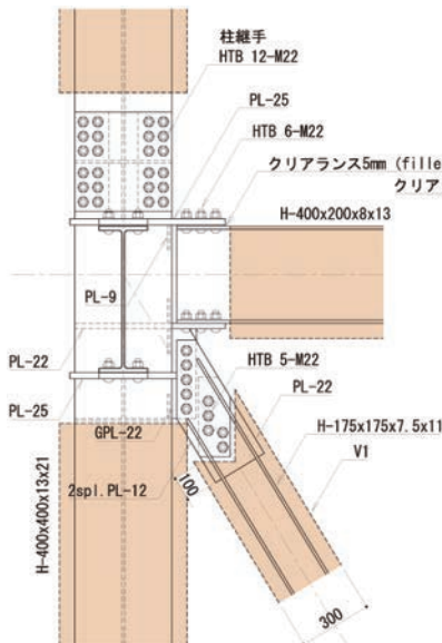
柱・桁ジョイント部詳細図
