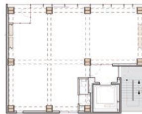
4～6階平面図
