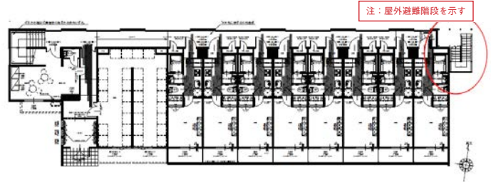
1階平面図
