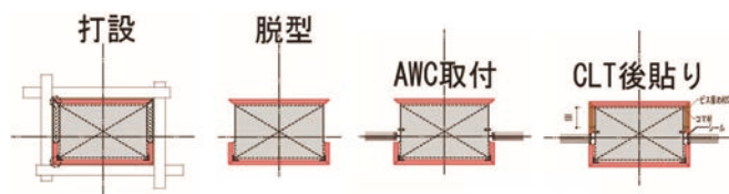
CLT 型枠による RC 造の木質化
