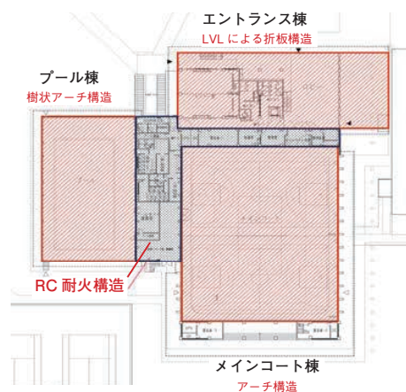
RC 造を介して 3 棟に分割
