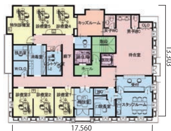
2階平面図
