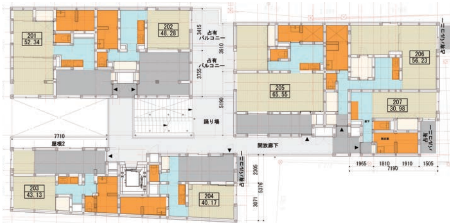
2階平面図
