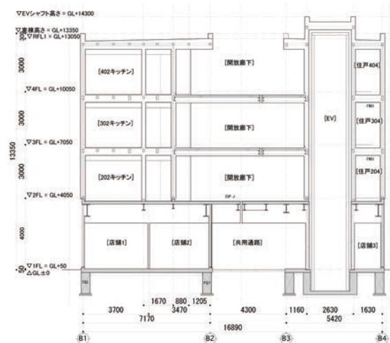
短手断面図
