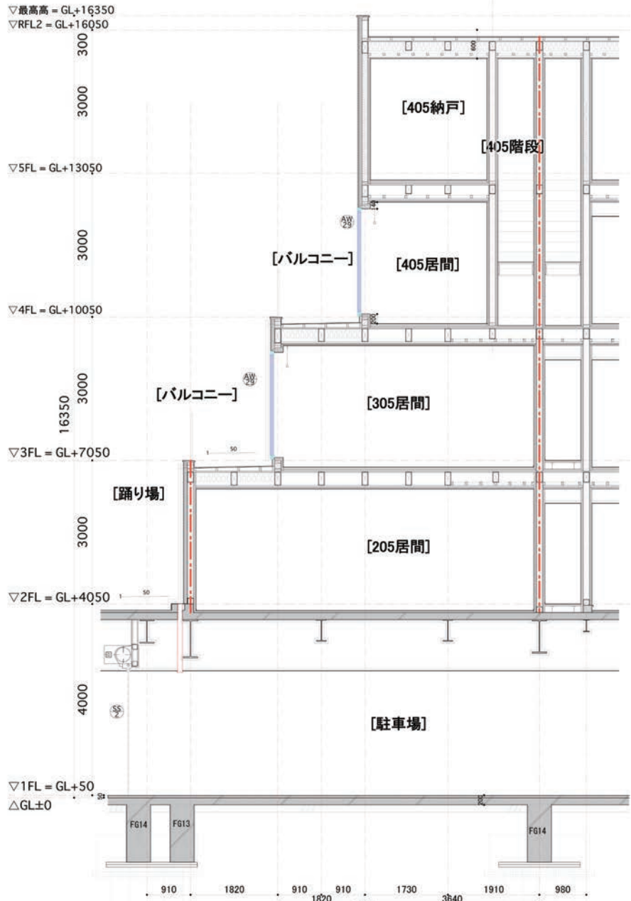
南棟矩計図
