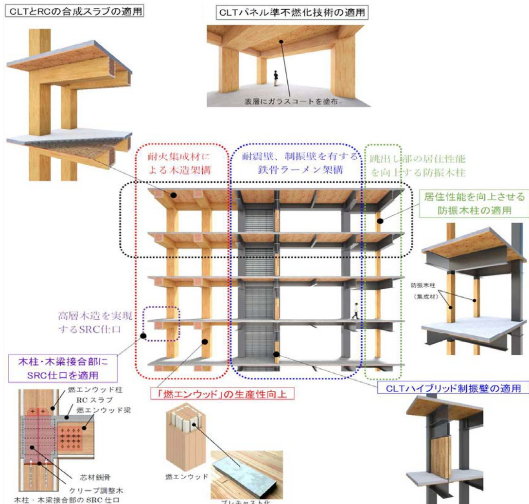
構造性能を向上しながら、木空間を創出する CLT 合成床
