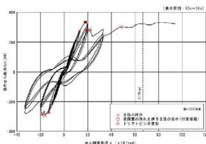
金物を使わない剛接仕口ユニット試験結果
