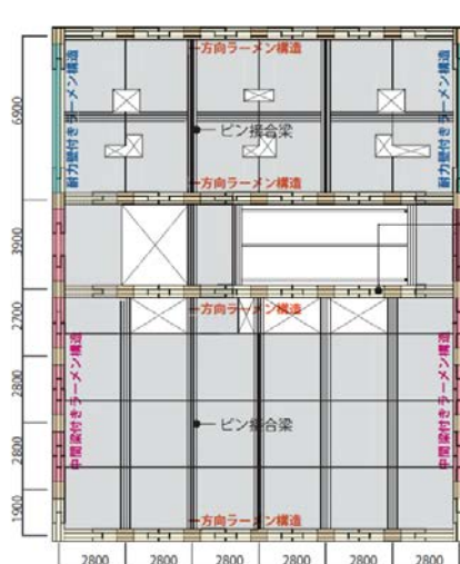
基準階伏図
