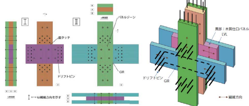
金物を使わない剛接十字仕口ユニットの構成
