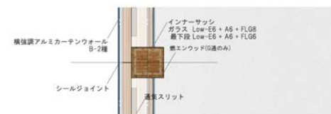
燃焼エンウッド部平面図
