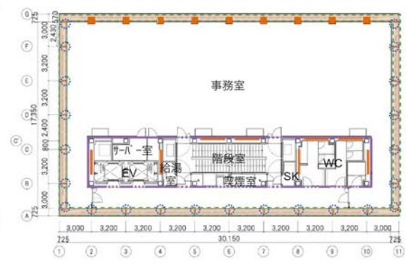
3～5階平面図
