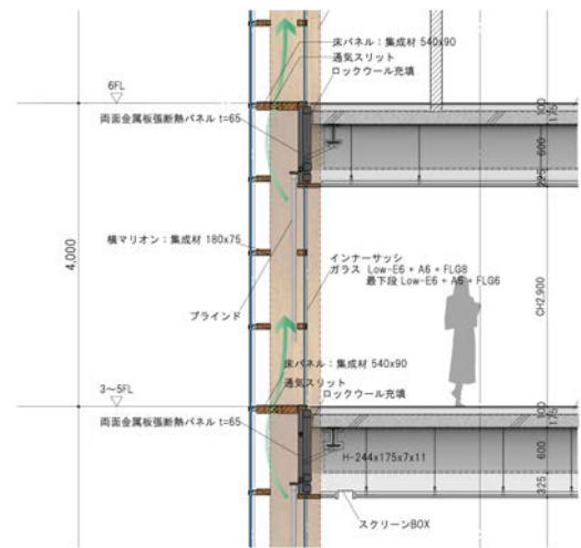
カーテンウォール部矩計図
