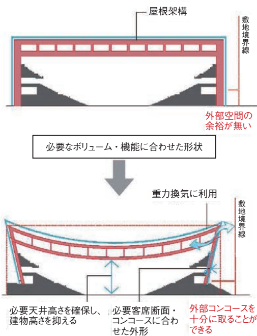
建物断面形状のイメージ図
