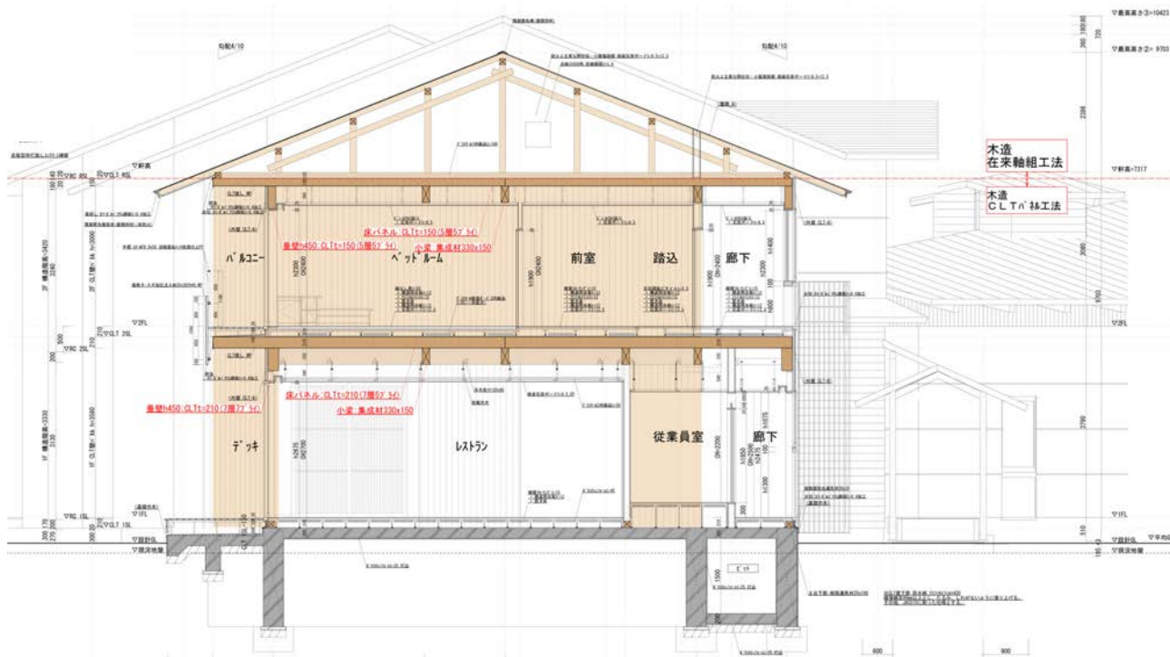
本館断面図
