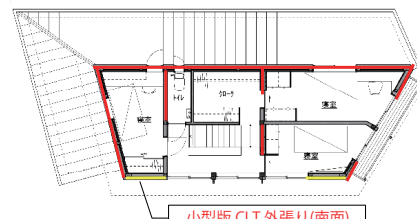
3 階平面図
