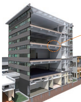
6 階建て以上の建物で 2 時間耐火となる床構造は国内初
