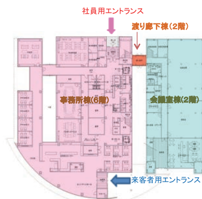
1 階平面図
