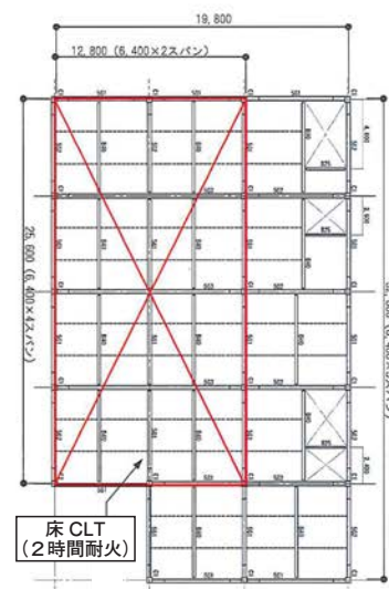
事務所棟 2 ～ 5 階床伏図
