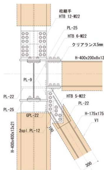
柱・桁ジョイント部詳細図
