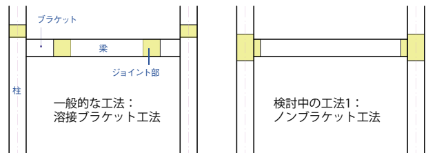
柱梁ジョイント工法の比較
