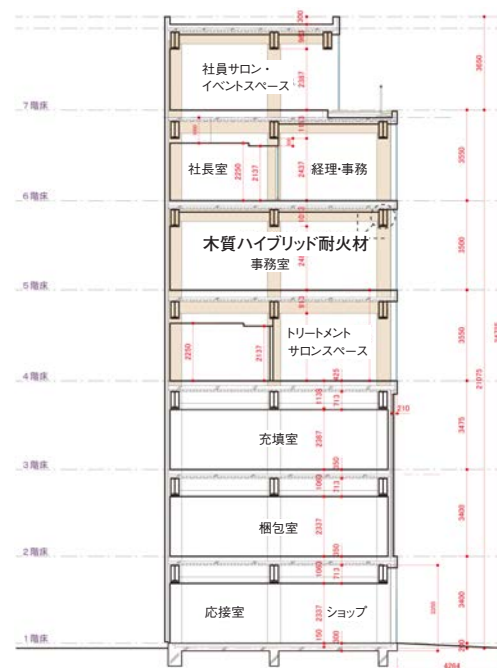
断面図
