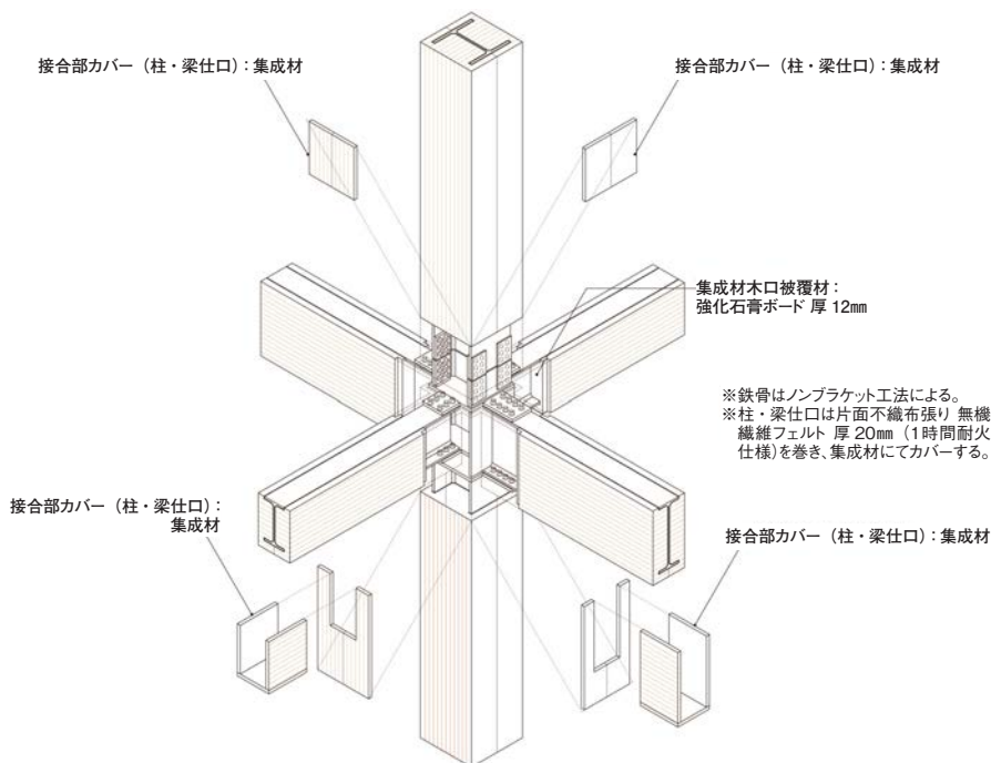
ノンブラケット工法の概要
