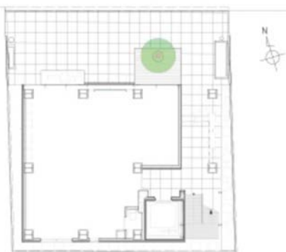
1階平面図
