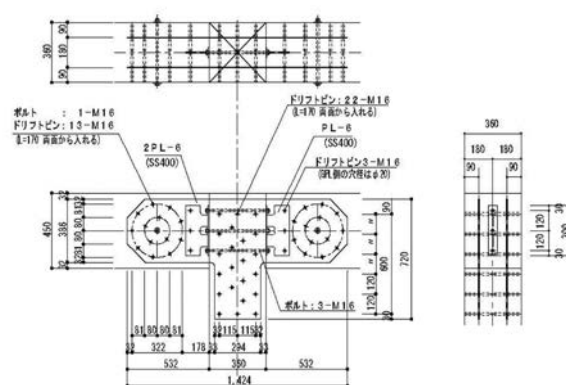
木質ラーメンの柱頭金物詳細
